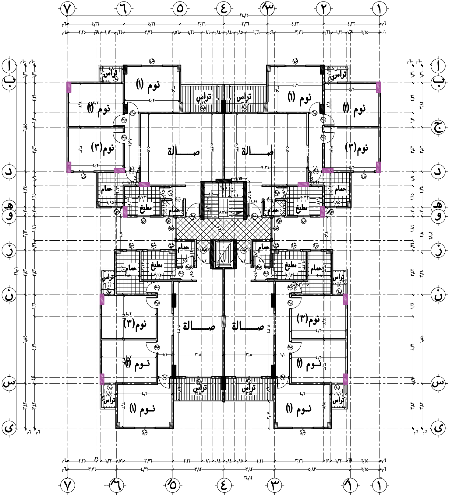
مسقط افقى للدور المتكرر
