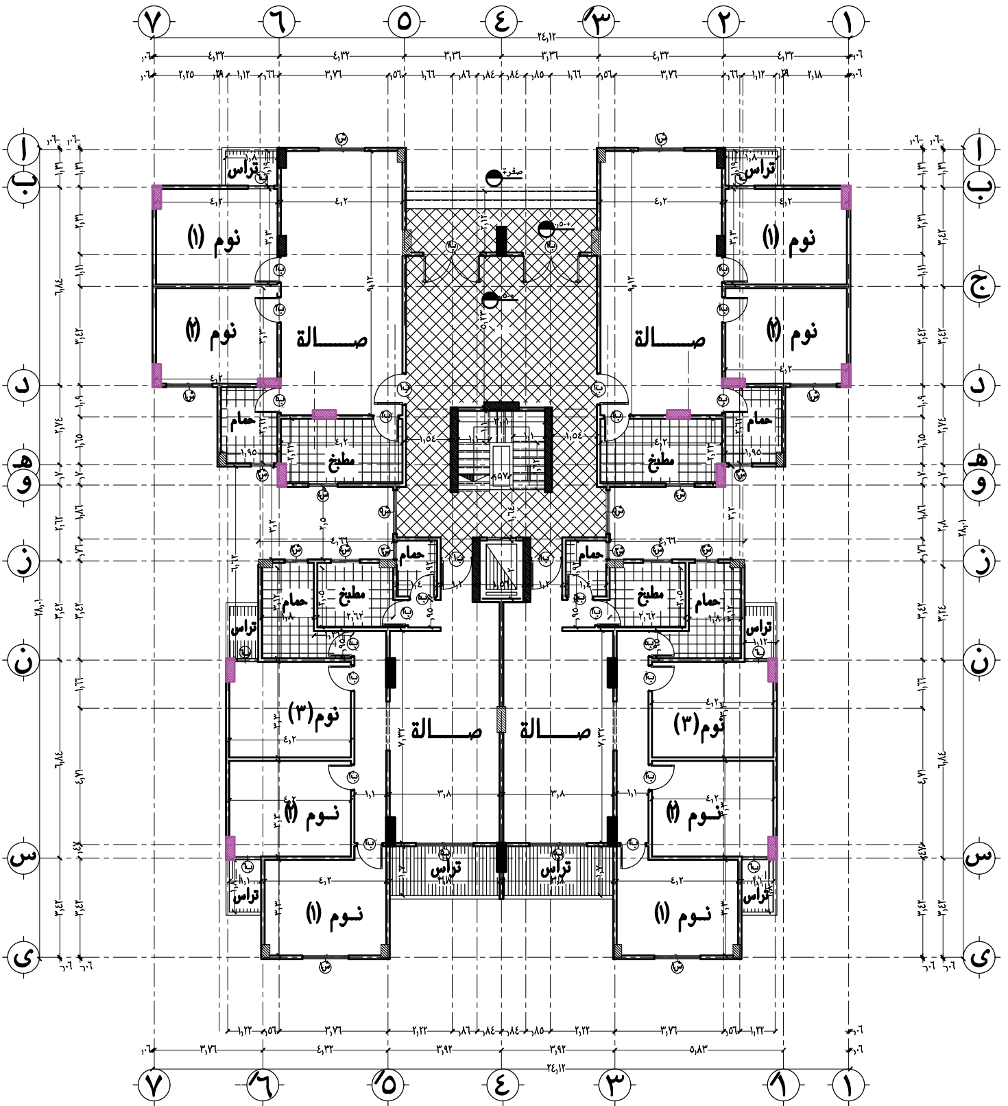
مسقط افقى للدور الارضى
