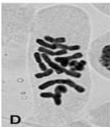
C-Mitosis
